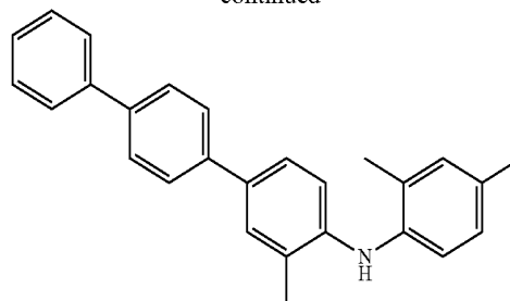
C 27 H 25 N Exact Mass: 363.20 Mol. Wt.: 363.49 C, 89.21; H, 6.93; Br, 3.85
